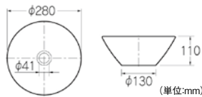
(単位:mm)
