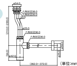
(単位:mm)
